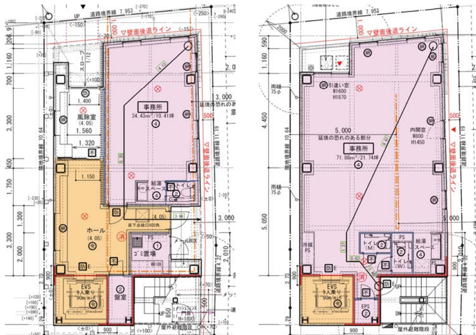
1階平面図
