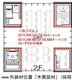
■ 外装材位置「木質部材」（採用部材は検討中） ■ 内装材位置「CLT材（60mm）」（間仕切り壁） ■ 内装材位置「CLT材（36mm）」
